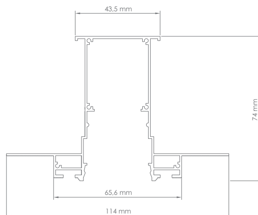
PROFILO DA INCASSO RECESSED PROFILE DA-CF-VELAR
