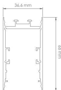
PROFILO ALUMINIUM PROFIL DA-PR-VELAR
